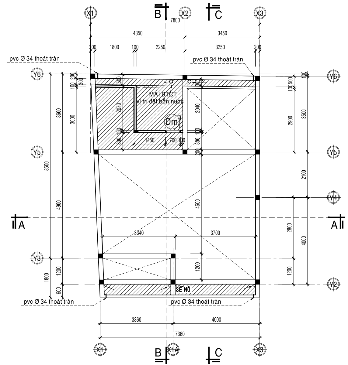
MẶT BẰNG MÁI SÊ NÔ...TL1/100
