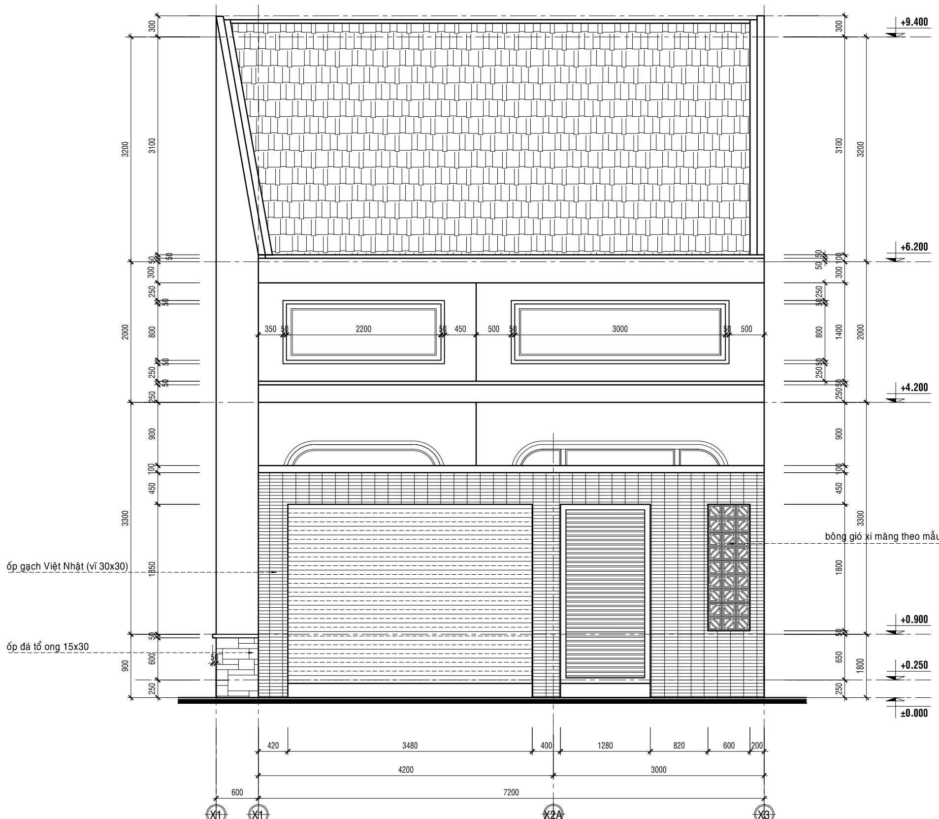
MẶT ĐỨNG X1-X3...TL1/ 50
