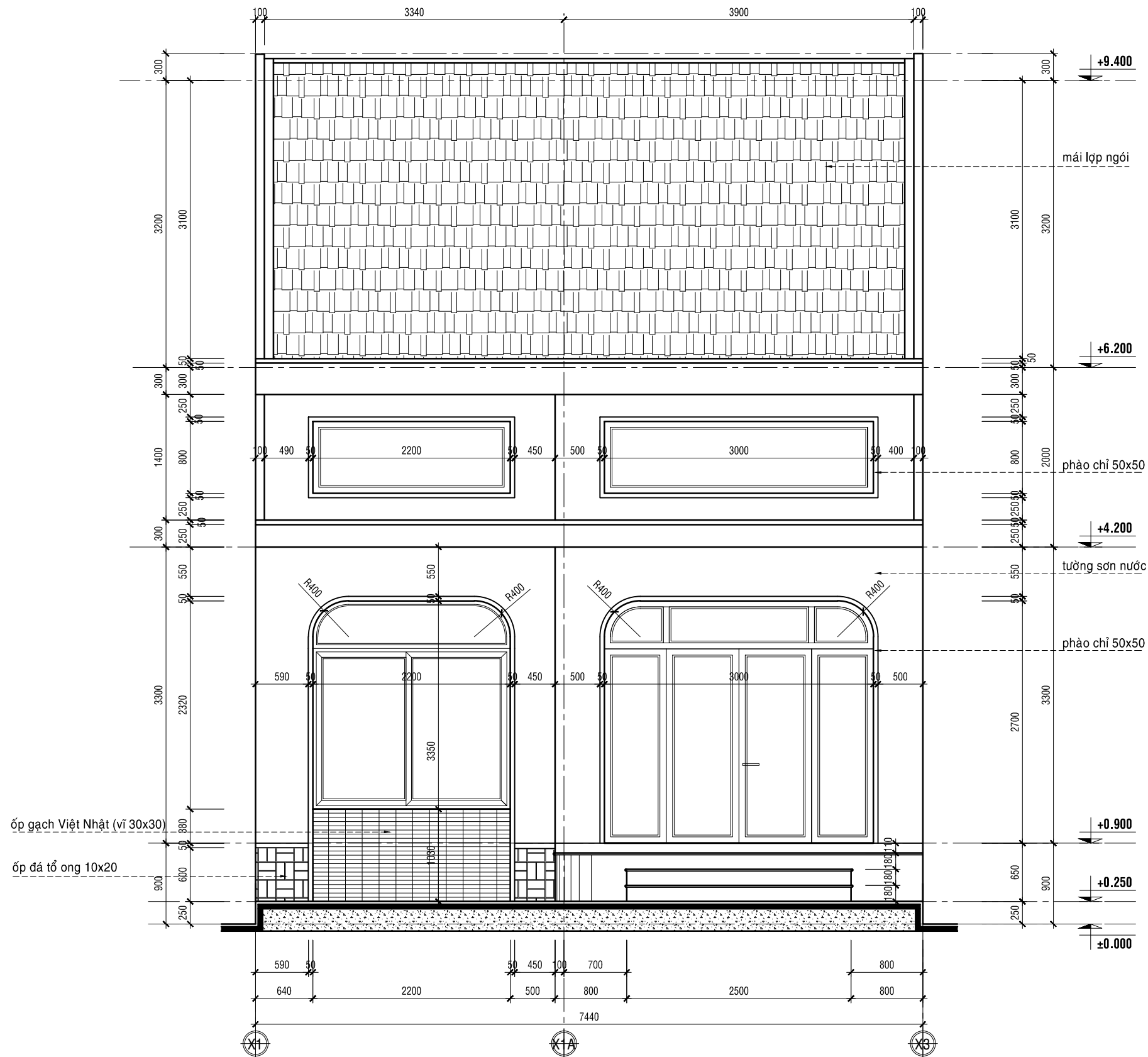
MẶT ĐỨNG X1-X3...TL1/ 50
